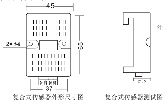
复合式传感器外形尺寸图
