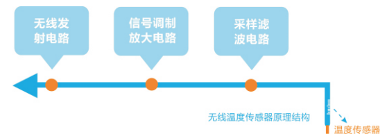
无源温度传感器原理结构图
