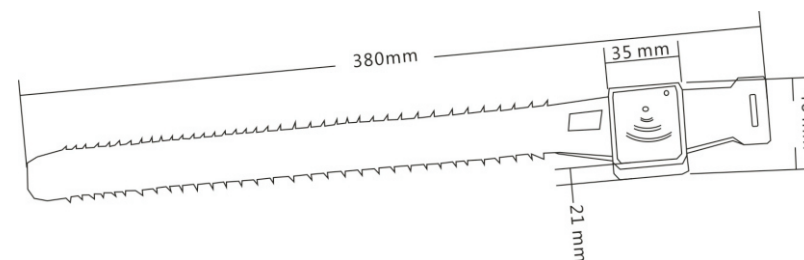
无线传感器表带外形尺寸 (单位: mm)
